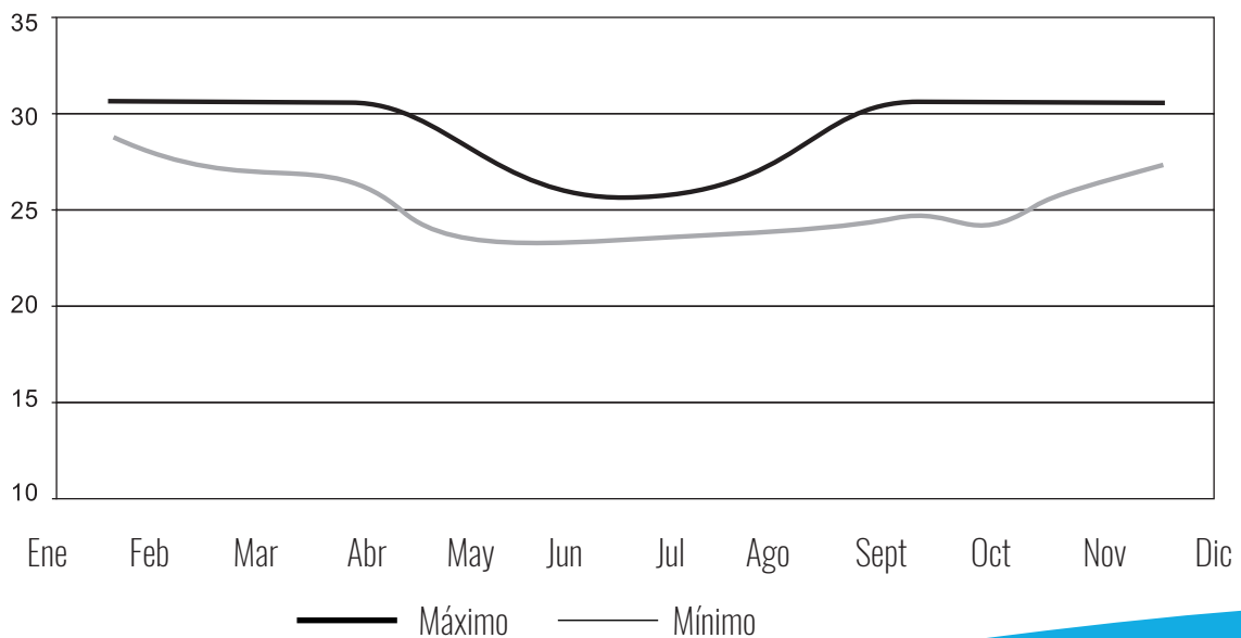
Rango Temperatura Piscina durante el período de operación en el día
